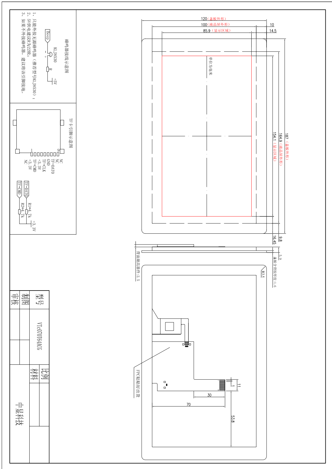
图 4 VTc070T64ACG 尺寸图
